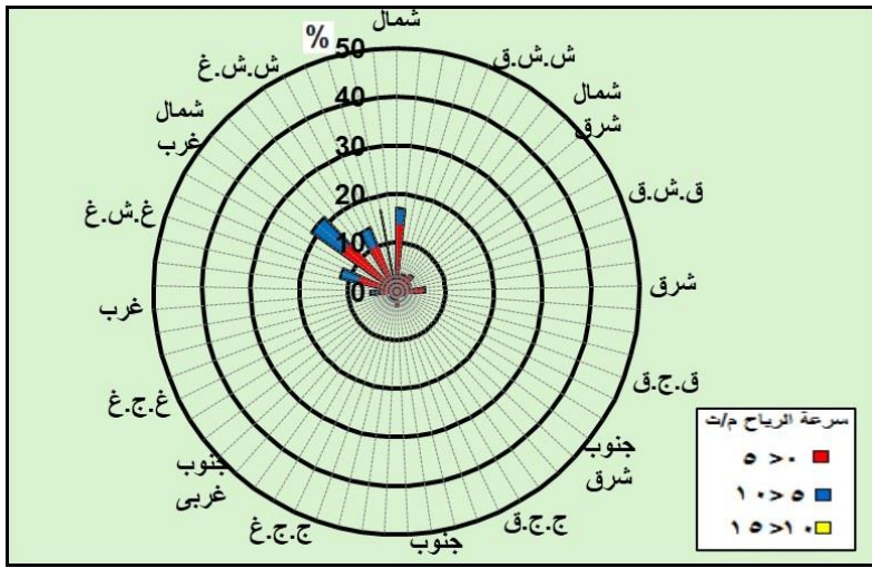
المصدر: مخرج تحليل بيانات سرعة الرياح واتجاتها خلال الفترة من من ( 2005 - 1976 ) بمحطة الضبعة شكل رقم (9) اتجاهات وسرعة الرياح المؤثرة بمنطقة الدراسة
